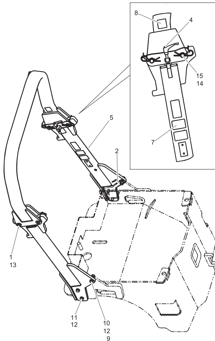
Diagrama de la estructura antivuelco
