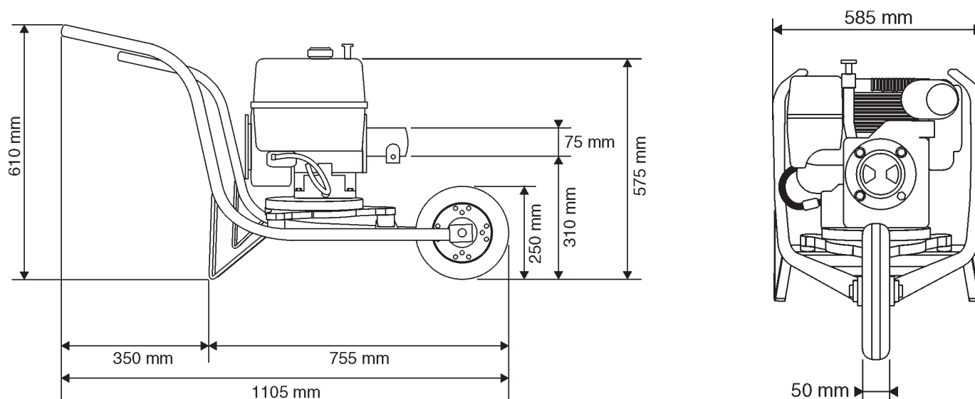
Figura 4. Unidad motriz tipo carretilla
