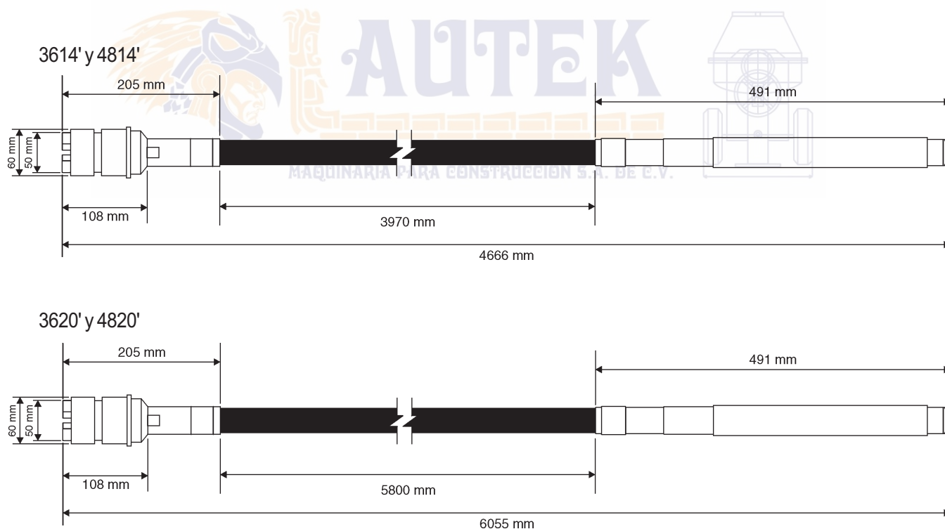
Figura 7. Dimensiones
