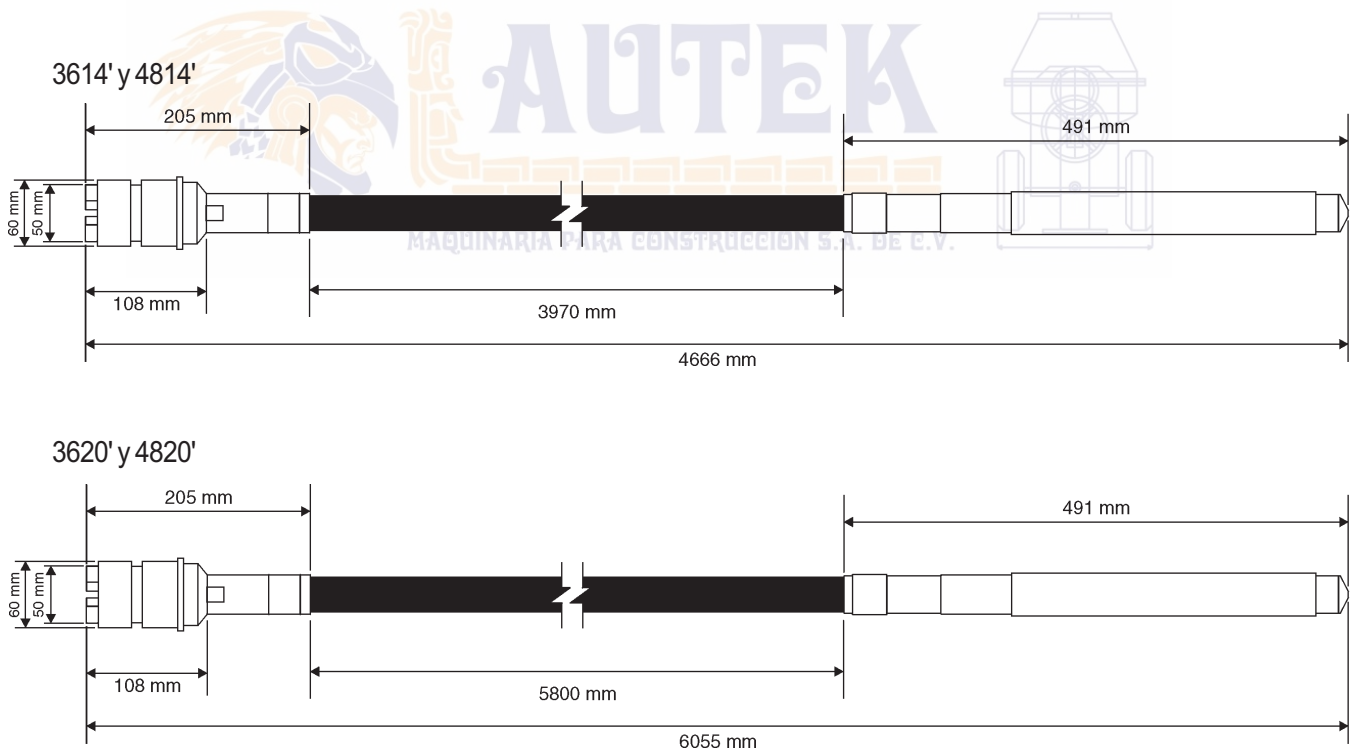
Figura 7. Dimensiones
